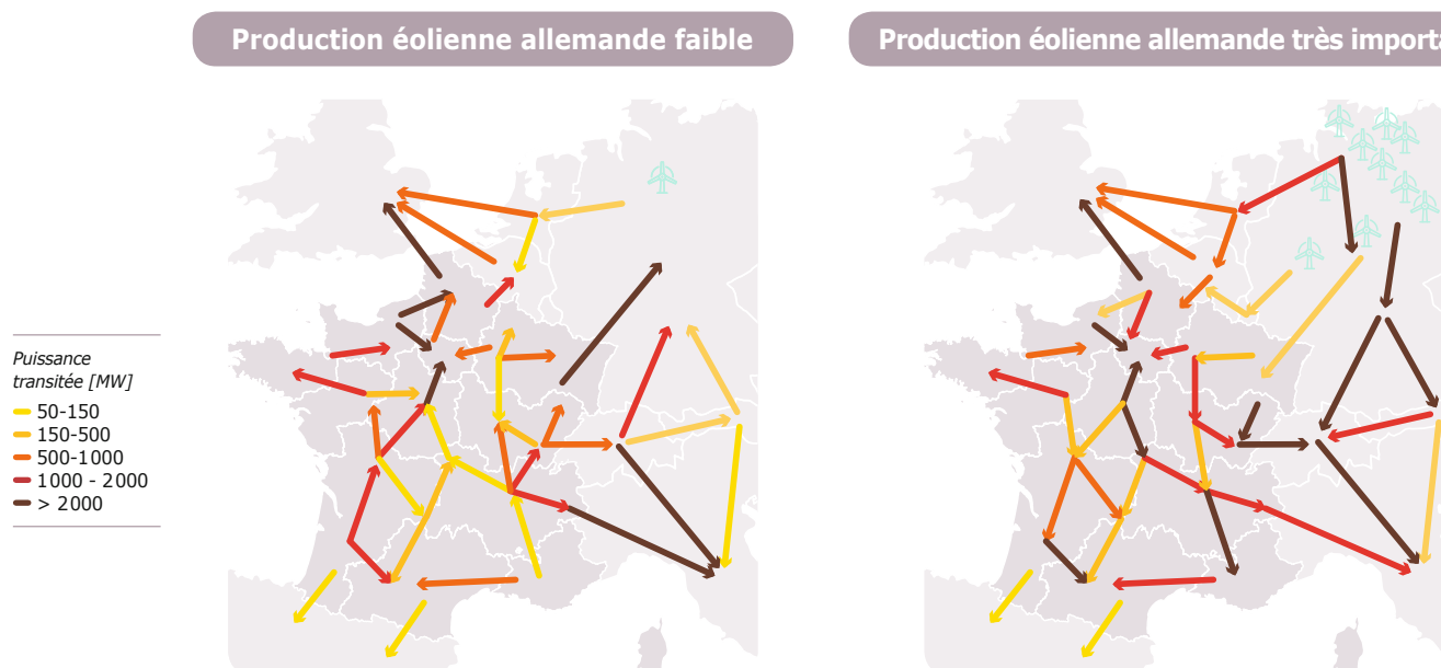
Figure 4. Influence de la production éolienne en Allemagne sur les flux sur le réseau en France
